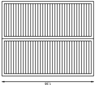
1 Malloquina practicable de dos hojas con lama fija. 1610x1980mm
