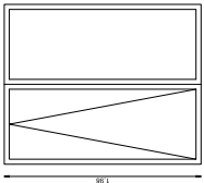
1 Puerta practicable de dos hojas una de ellas oscilobalante. 1610x1980mm
