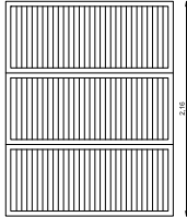
4 Malloquinas practicables de tres hojas con lama fija. 2160x1680mm
