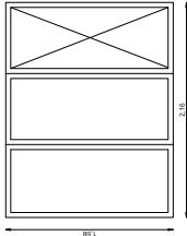
4 Ventanas de dos hojas practicables con fijo lateral. 2160x1680mm
